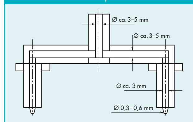
Abbild. 6.1.3 · Heißkanalsystem für kleine Bauteile
