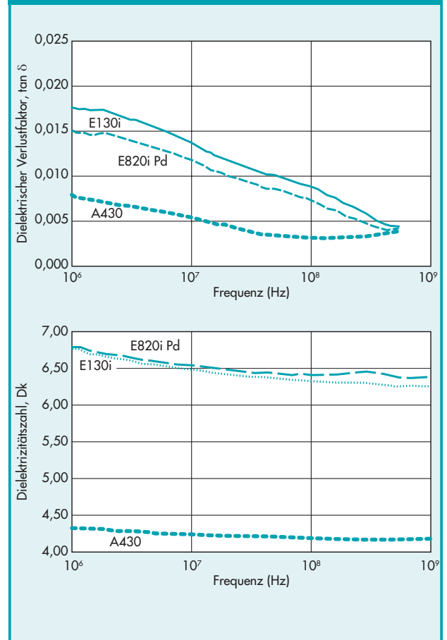
Abbild. 3.4.2 · Frequenzabhängigkeit der Dk/tan δ-Werte einiger Vectra®-Typen (Gold bedampft)
