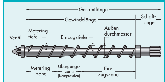
Abbild. 6.1.1 · Dreizonenschnecke für die Verarbeitung von Vectra® LCP
