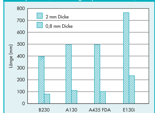
Abbild. 8.1.1 · Fließweglängen (Einspritzdruck: 195 bar hydraulisch/ca. 1.000 bar spezifisch, Werkzeugtemperatur: 100°C)
