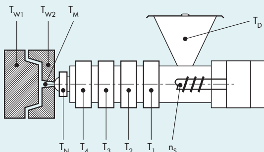
Abbild. 6.2.1 · Verarbeitungsbedingungen
