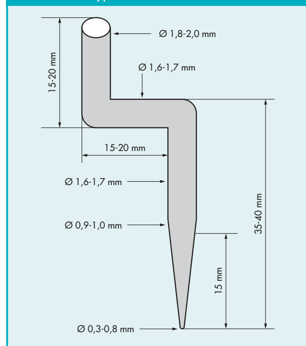
Abbild. 8.2.1 · Typischer Verteilerkanal für Vectra® LCP
