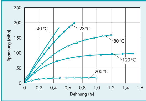
Abbild. 3.1.8a · Einfluss der Temperatur auf das Spannungs-Dehnungs-Verhalten, Zugversuch, Vectra® B230
