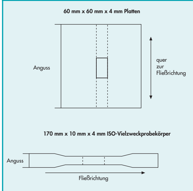
Abbild. 3.2.5 · Prüfkörper für Messung des Längenausdehnungskoeffizienten
