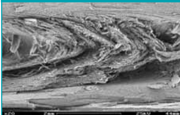
Abbild. 3.0 · Bruchfläche von unverstärktem Vectra®
