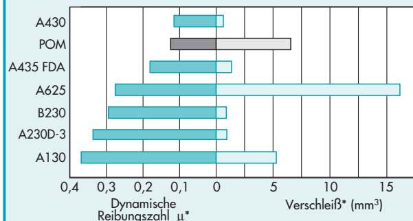
Abbildung 3.1.15 · Reibung und Verschleiß
