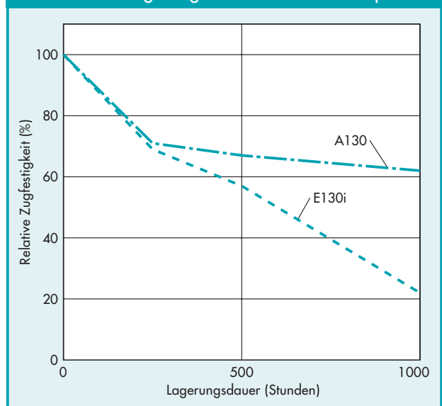
Abbild. 4.1.3 · Zugfestigkeit in Abhängigkeit von der Lagerungsdauer in Wasserdampf
