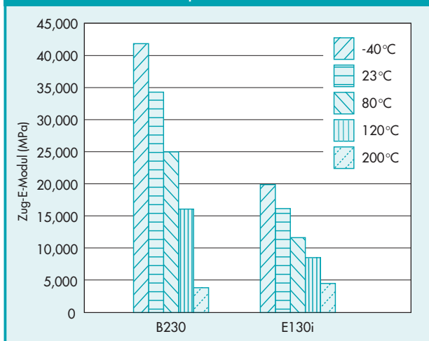
Abbild. 3.1.9 · Zug-E-Modul in Abhängigkeit von der Temperatur, Vectra® LCP
