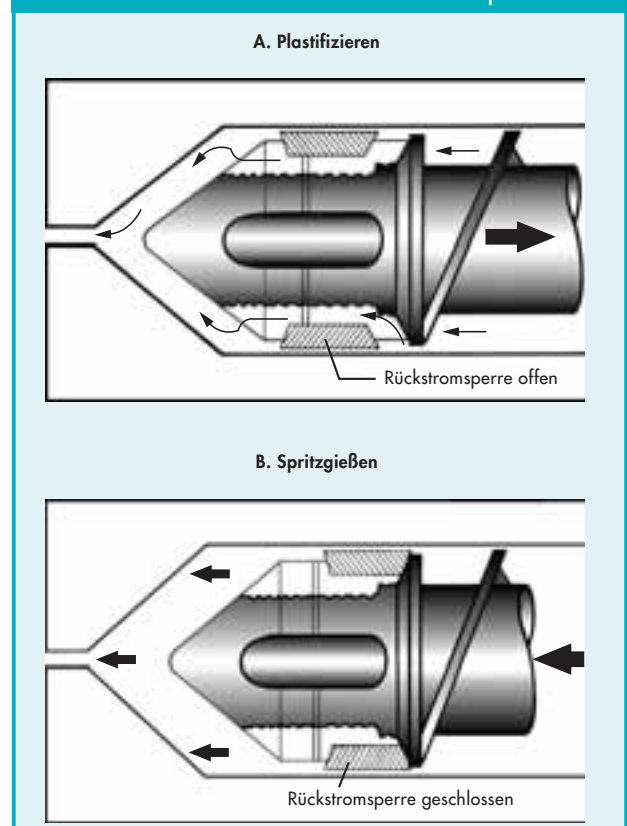
Abbild. 6.1.2 · Funktion des Rückstromsperrventils
