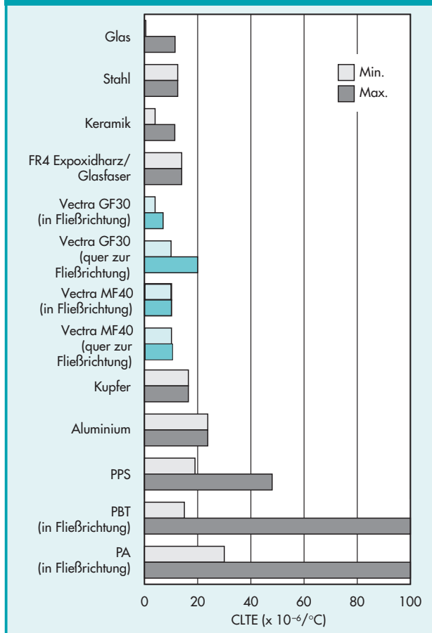
Abbild. 3.2.4 · Lineare Wärmeausdehnungskoeffizienten von ausgewählten Werkstoffen
