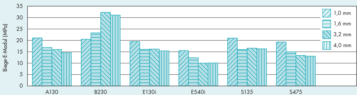
Abbild. 3.1.5 · Biege-E-Modul in Abhängigkeit von der Wanddicke bei Vectra®
