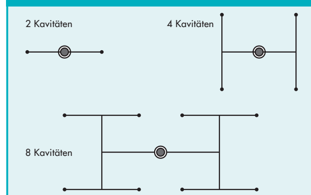
Abbild. 6.1.4 · Heißkanalverteiler
