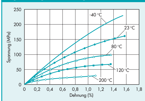
Abbild. 3.1.8b · Einfluss der Temperatur auf das Spannungs-Dehnungs-Verhalten, Zugversuch, Vectra® E130i
