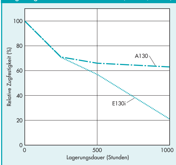
Abbild. 4.1.1 · Zugfestigkeit in Abhängigkeit von der Lagerungsdauer in heißem Wasser (120°C, 2 bar)
