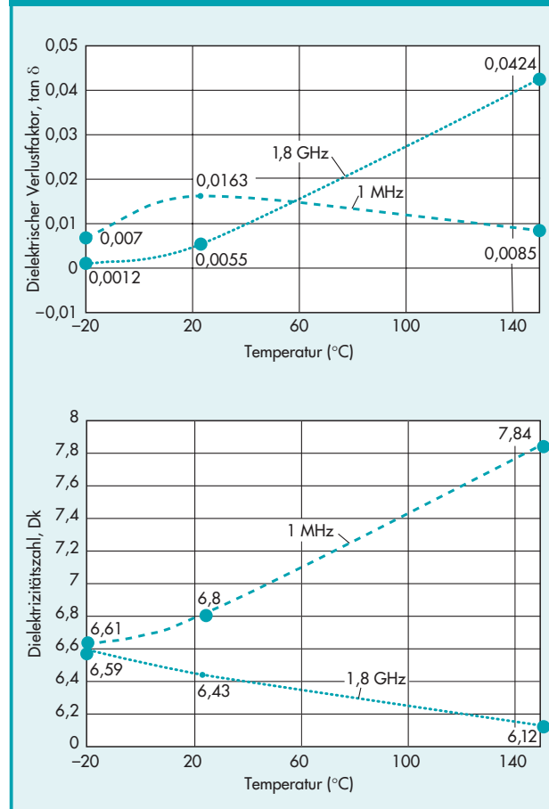
Abbild. 3.4.1 · Temperaturabhängigkeit der Dk/tan δ-Werte von Vectra® E820i Pd (Gold bedampft)
