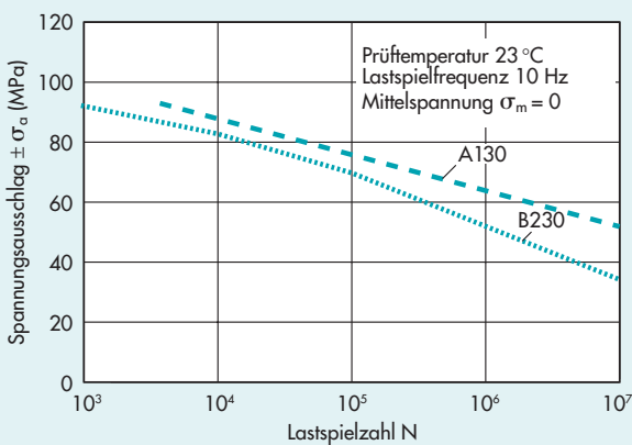
Abbildung 3.1.14 · Wöhler-Kurven für Vectra, ermittelt in Fließrichtung im Dauerschwingversuch
