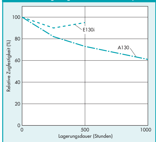
Abbild. 4.1.4 · Zug-E-Modul in Abhängigkeit von der Lagerungsdauer in Wasserdampf
