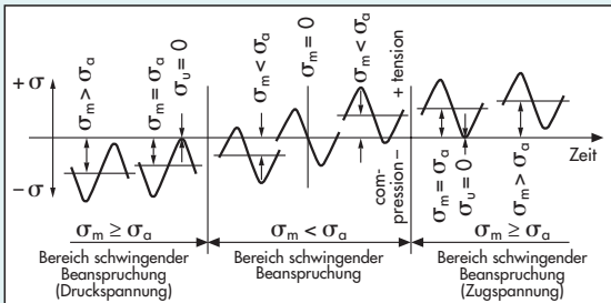
Abb. 3.1.13 · Beanspruchungsbereiche im Dauerschwingversuch
