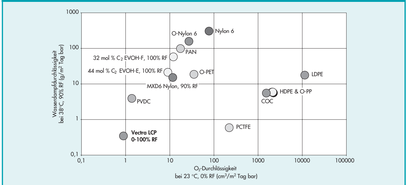
Abbild. 4.3.1 · Durchlässigkeit verschiedener Polymerfolien (Folienstärke 25 µm)
