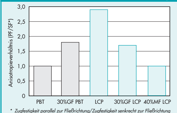
Abbild. 3.1.1 · Anisotropievergleich* zwischen Vectra® LCP und Celanex PBT (ISO Universal-Probekörper)
