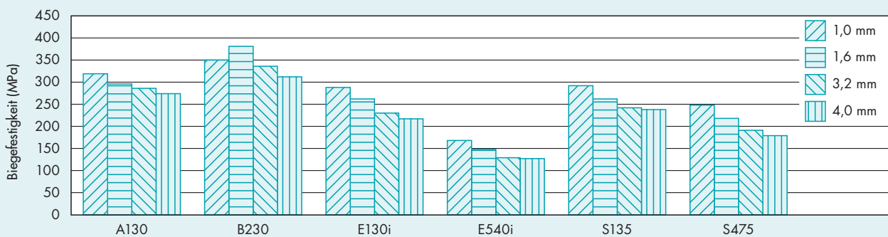
Abbild. 3.1.6 · Biegefestigkeit in Abhängigkeit von der Wanddicke bei Vectra®
