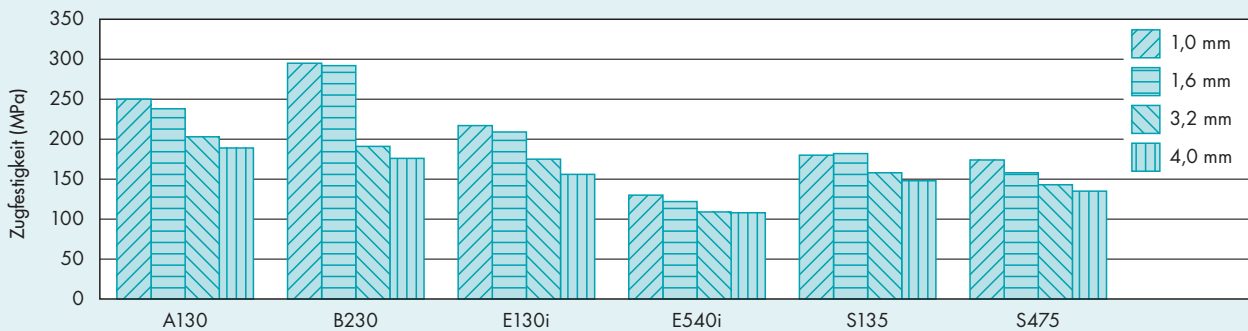
Abbild. 3.1.4 · Zugfestigkeit in Abhängigkeit von der Wanddicke bei Vectra®
