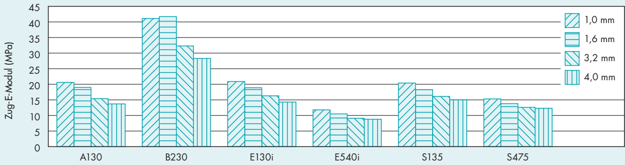
Abbild. 3.1.3 · Zug-E-Modul in Abhängigkeit von der Wanddicke bei Vectra®
