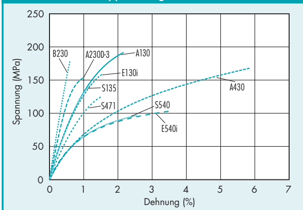
Abbild. 3.1.7 · Spannungs-Dehnungskurven einiger Vectra-Typen, Zugversuch, 23°C
